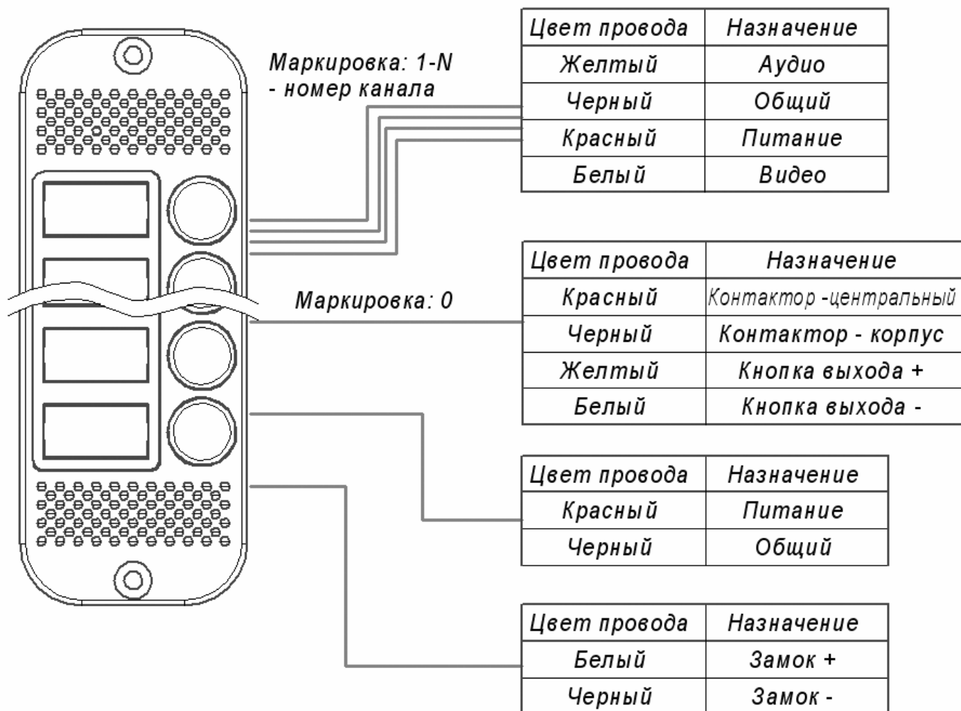
Рис.2 Схема подключения панели.
