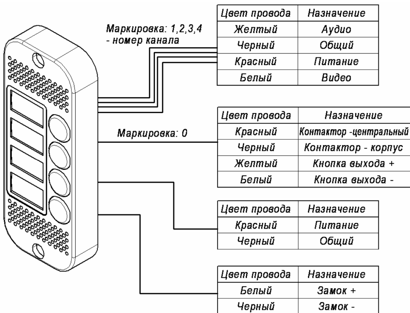
Рис.2 Схема подключения панели.
