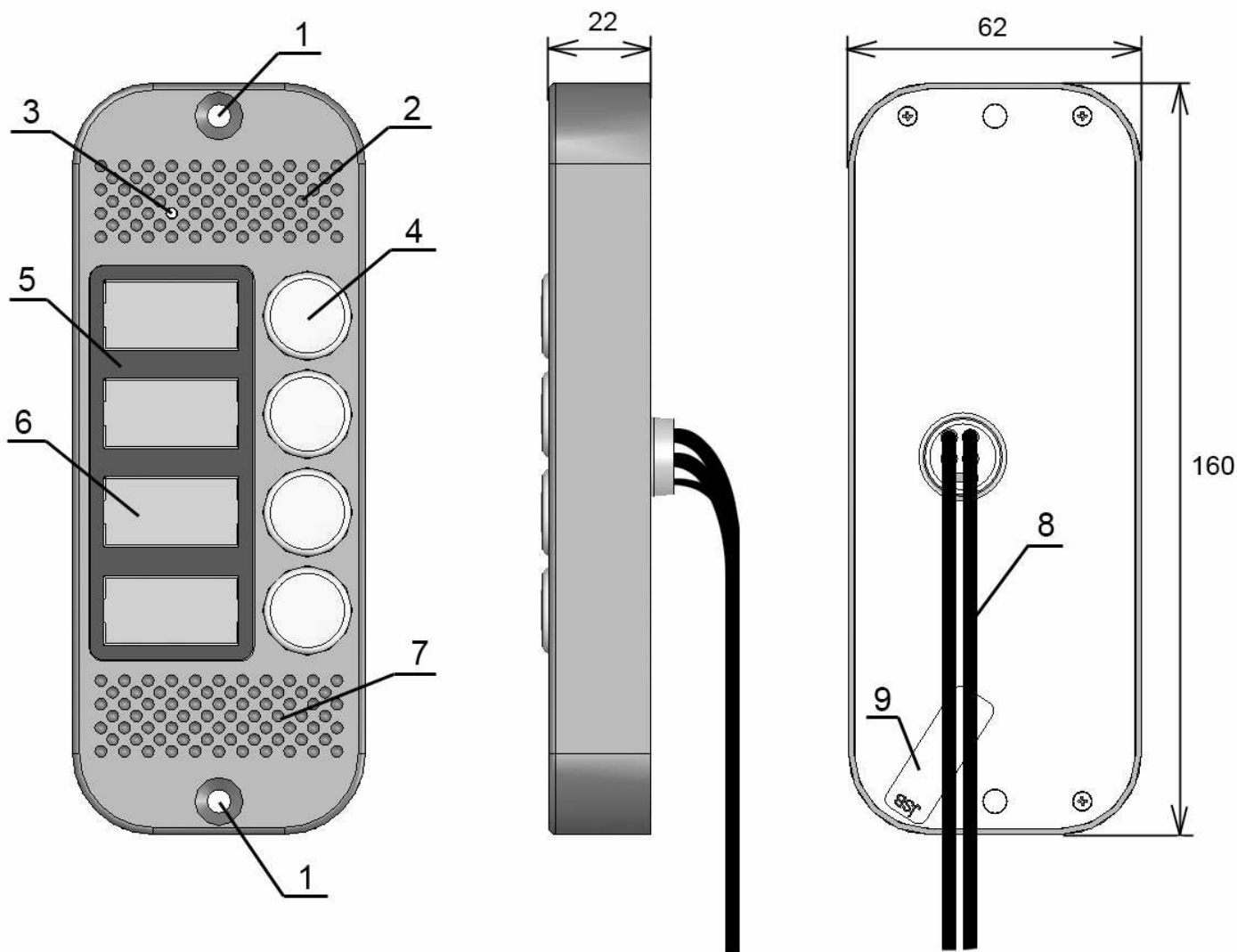
Рис. 1. Назначение основных узлов панели: 1- Места крепления панели (закрываются заглушками). 2- Зона микрофона со скрытой прорезью. 3- Видеокамера. 4- Кнопки вызова абонентов. 5- Защитный фильтр инфракрасной подсветки. 6- Места для обозначения абонентов (подсвечиваются, закрываются защитными стеклами),. 7- Зона динамика со скрытыми прорезями. 8- Провода подключения (назначение см. ниже). 9- Гарантийная пломба.
